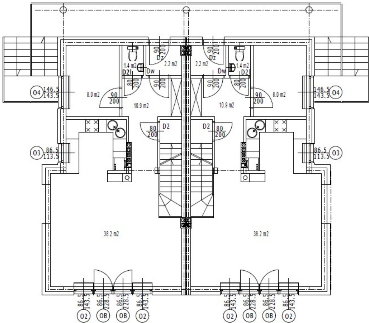
rzut parteru
